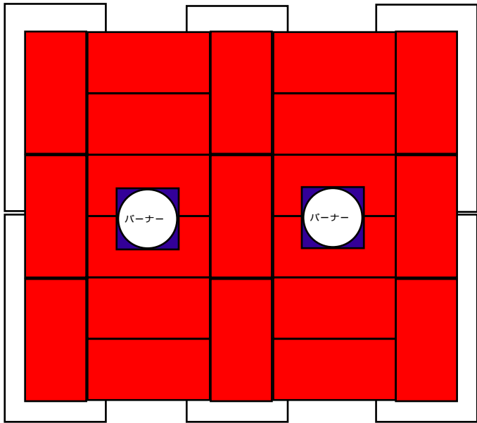
1階層 (コンクリートブロック) 2階層 (バーナータイル+耐火煉瓦)
