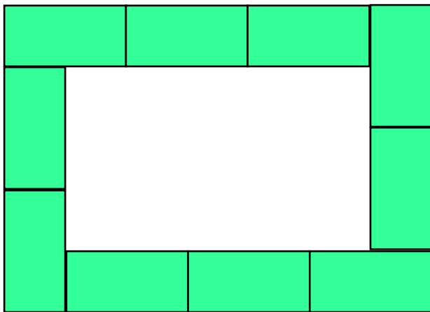
1階層 (コンクリートブロック) 2階層 (バーナータイル+耐火煉瓦)
